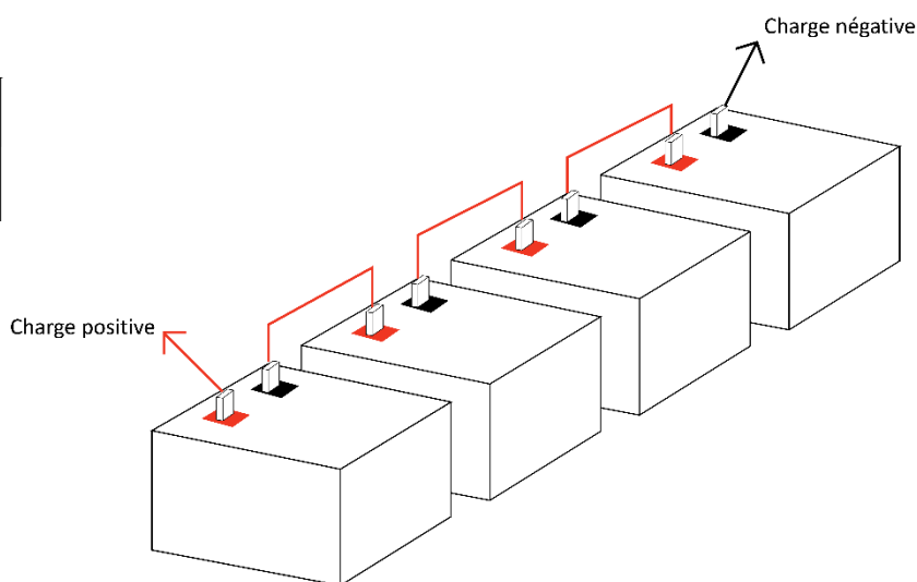
Figure 4.2 : Quatre batteries 8D connectées en série pour créer une banque de batteries 48V 270Ah
